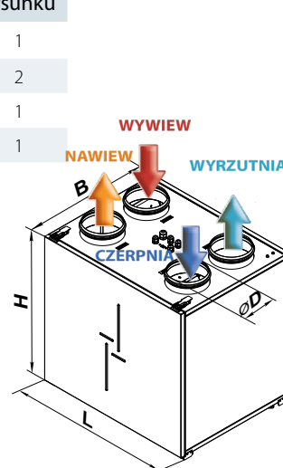
RYS.1. VUT/VUE 160/350/550 VB EC
