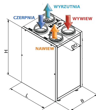
RYS.2. VUT(E) 250 VB EC L/R
